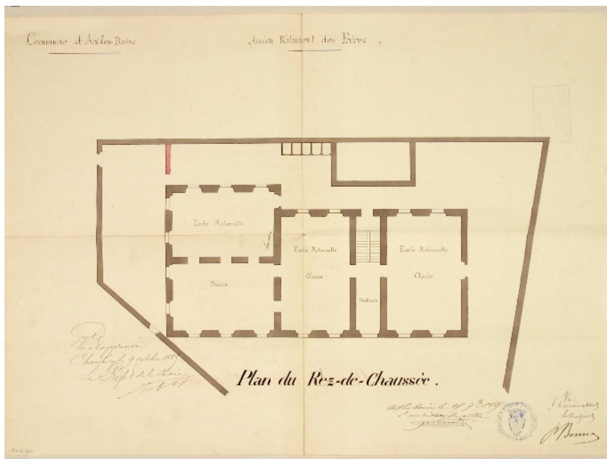
Plan du rez-de-chaussée, 1885
