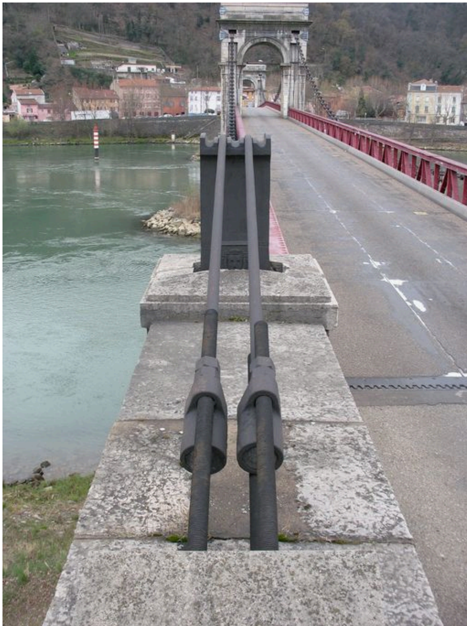
Câble porteur, vue partielle : massif d'ancrage et support (depuis la rive gauche)
