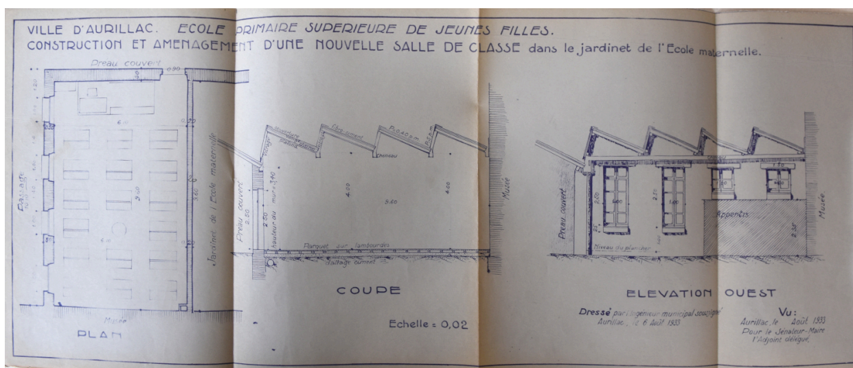
Plan, coupe et élévation de la nouvelle salle de classe dans le jardin de l'école maternelle, 1933 (AD Cantal, E DEP 1500/1487)
