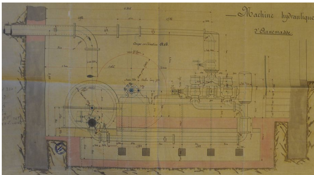
Coupe transversale de la machine hydraulique. Plan. Archives municipales d'Annemasse © Archives municipales d'Annemasse. 36/36
