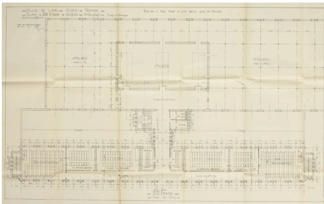
Ecole de tissage. Plan du 2e étage au niveau des ateliers, cours du jour, Lyon le 9/06/1927, Tony Garnier. (AC Lyon. 511 WP 003)
