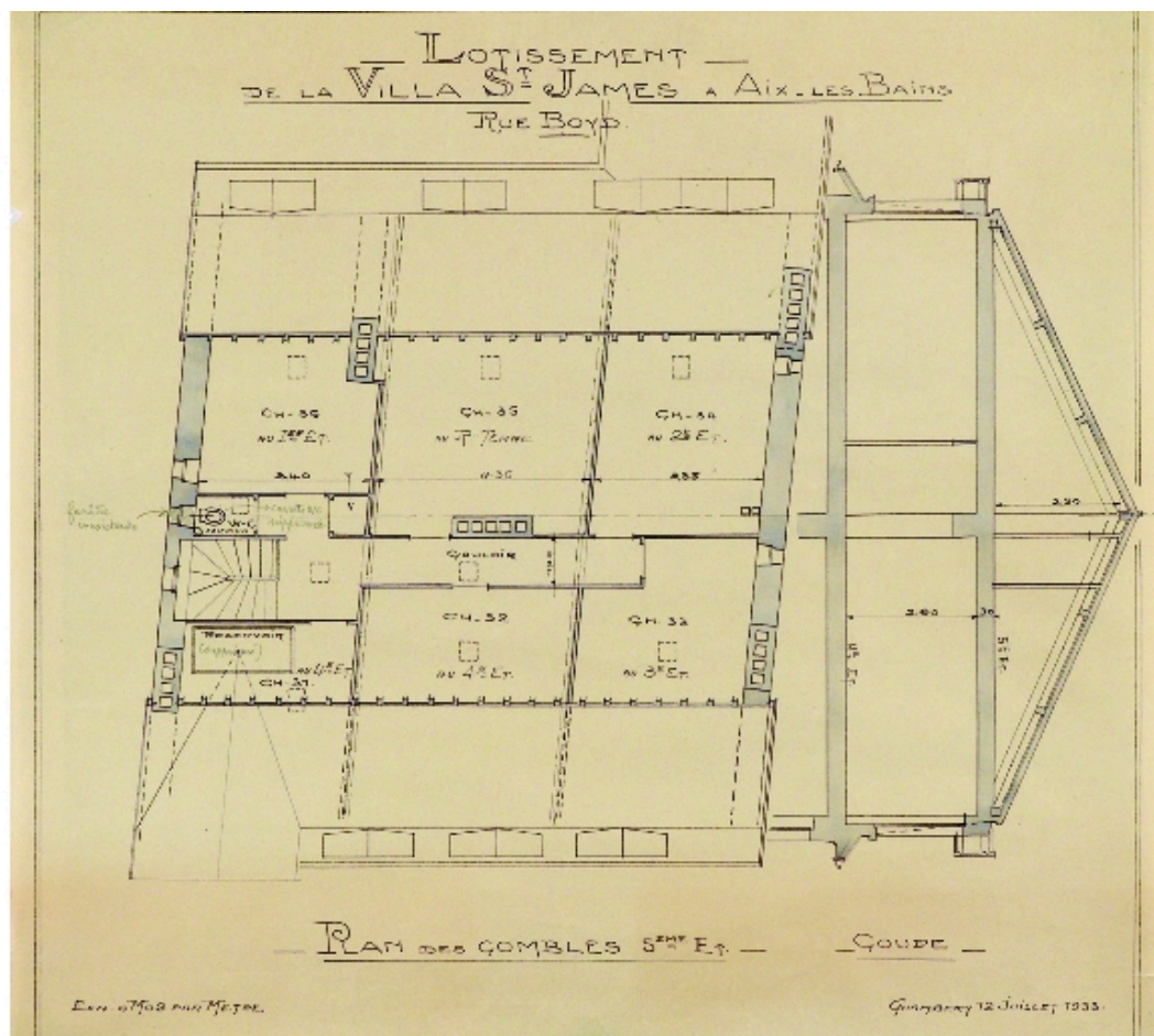
Plan et coupe de l'étage de combles
