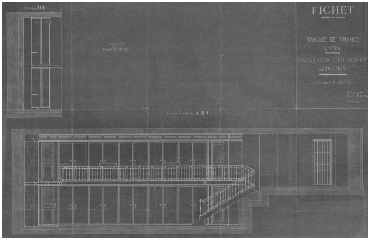
Coupe sur la salle des coffres aménagée par Fichet (1922) (Banque de France, service du Patrimoine Historique et Artistique, non coté, dessin de la maison Fichet).
