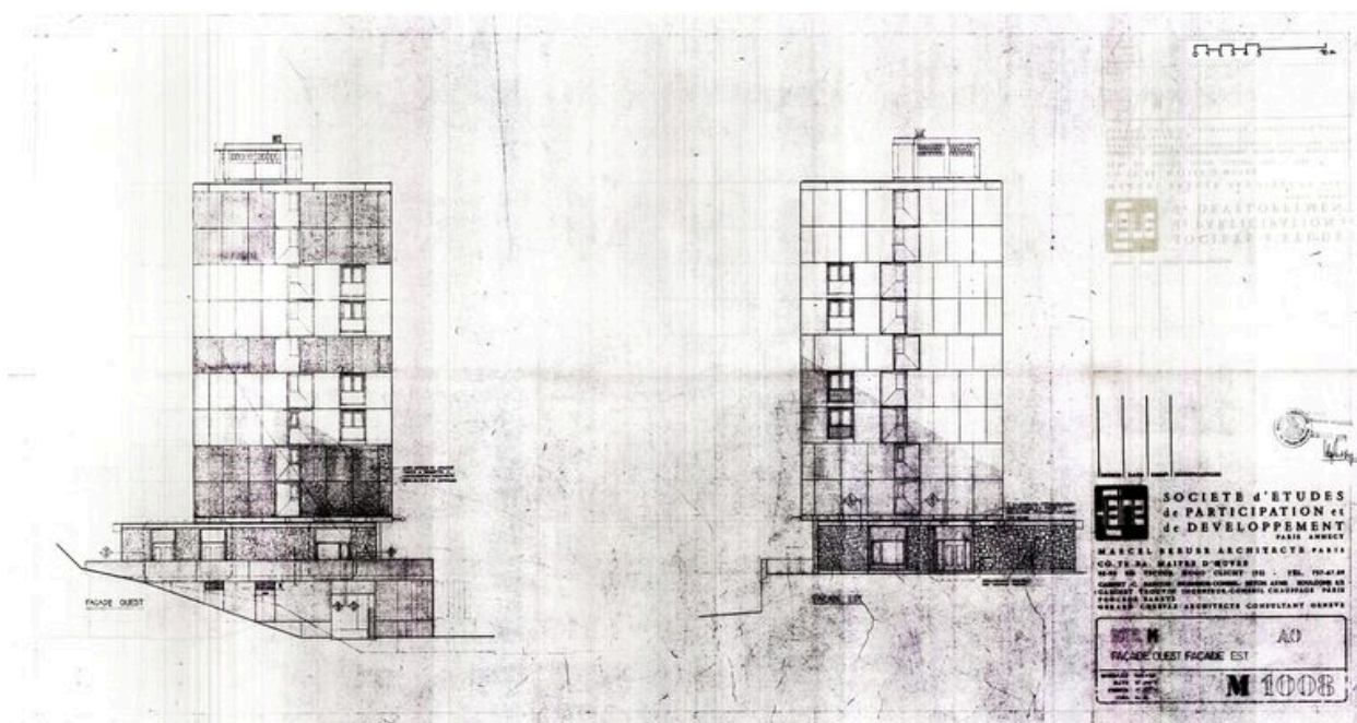
Hôtel M. Elévations ouest et est. Marcel Breuer architecte, 27 janvier 1971 (AC Arâches-la Frasse)
