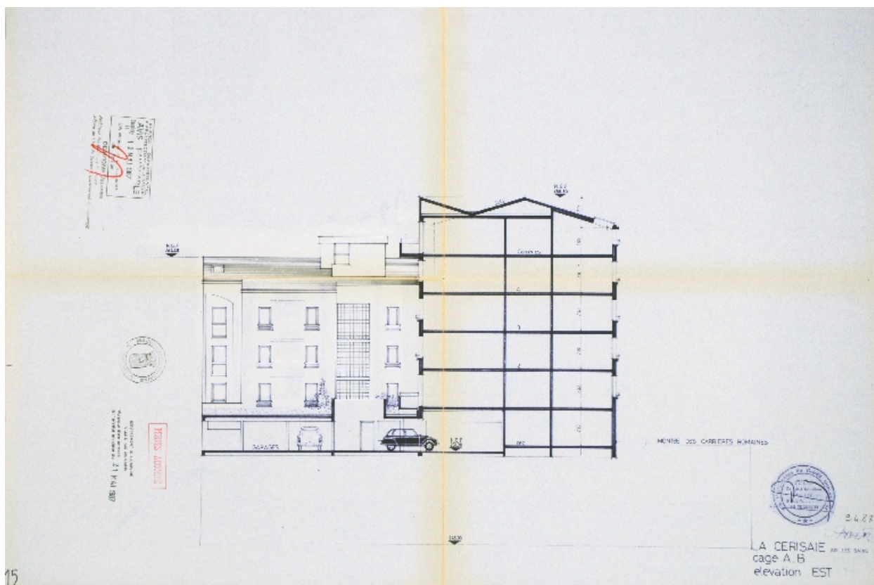
Élévation est et coupe
