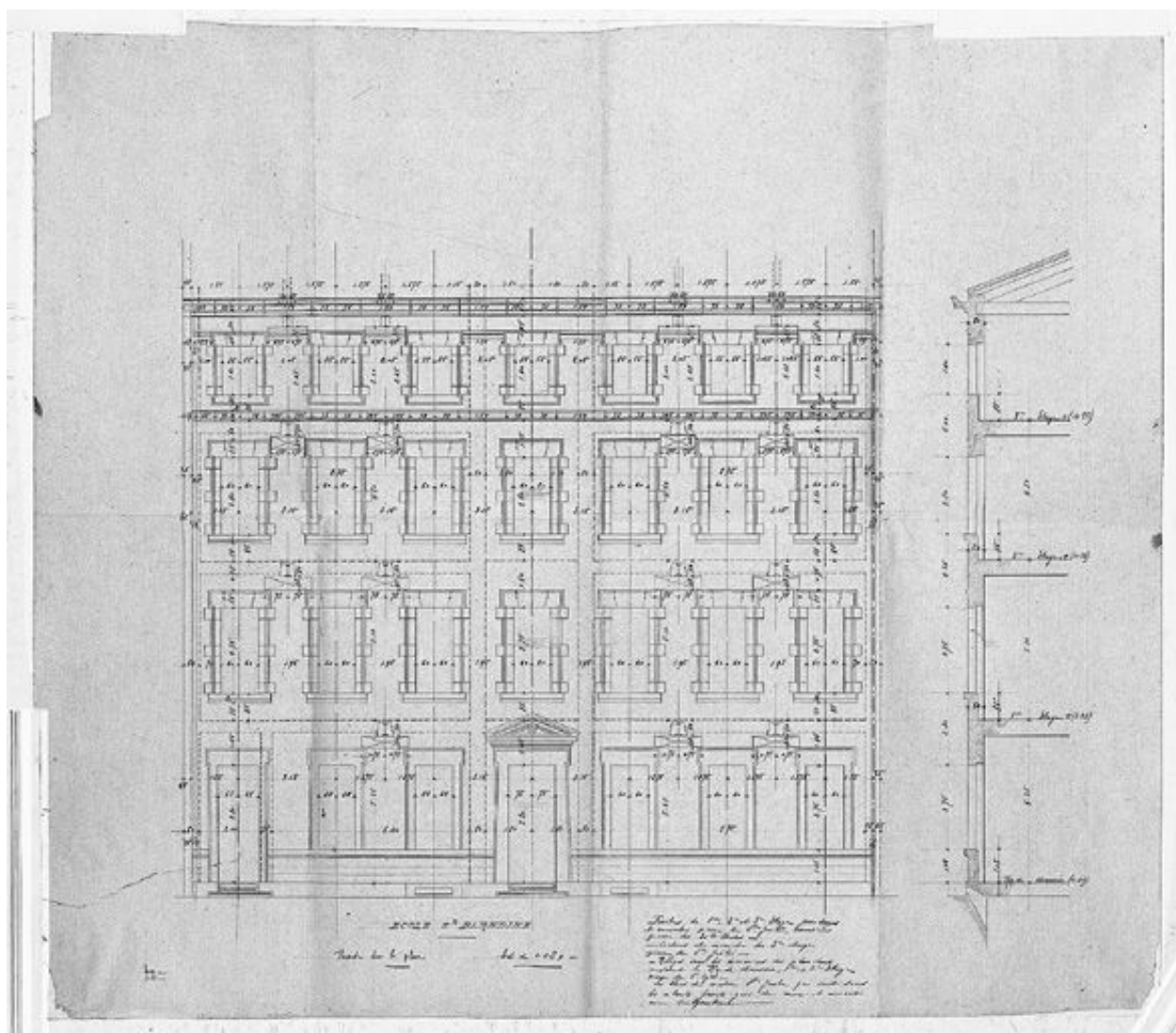
Elévation ouest cotée
