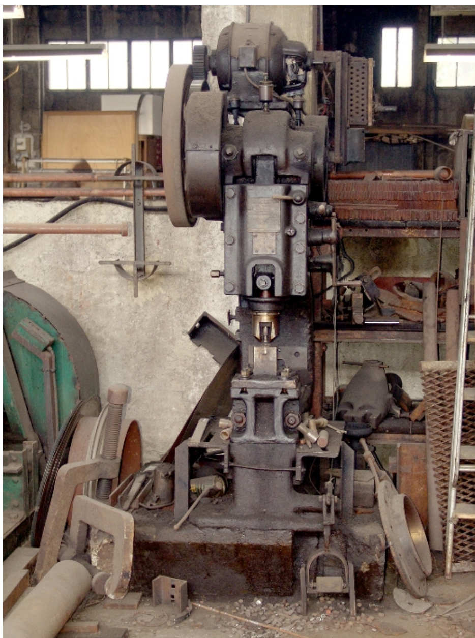
Machine-outil : cisaille
