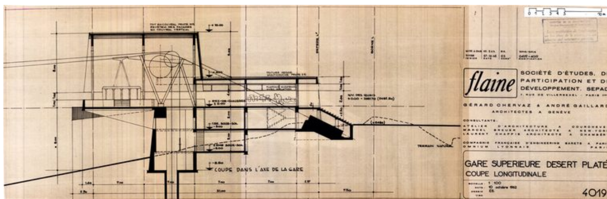
Coupe longitudinale. Gérard Chervaz et André Gaillard architectes, 10 octobre 1962. Modifié les 27 octobre 1962 et 22 octobre 1963 (AC Magland)
