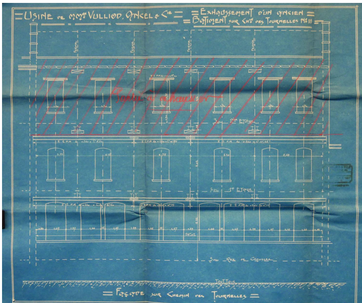
Façade, exhaussement d'un bâtiment 1912, usine Vulliot-Ancel (AC Lyon 314W461-468)
