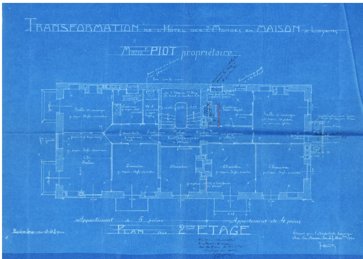
Plan du second étage
