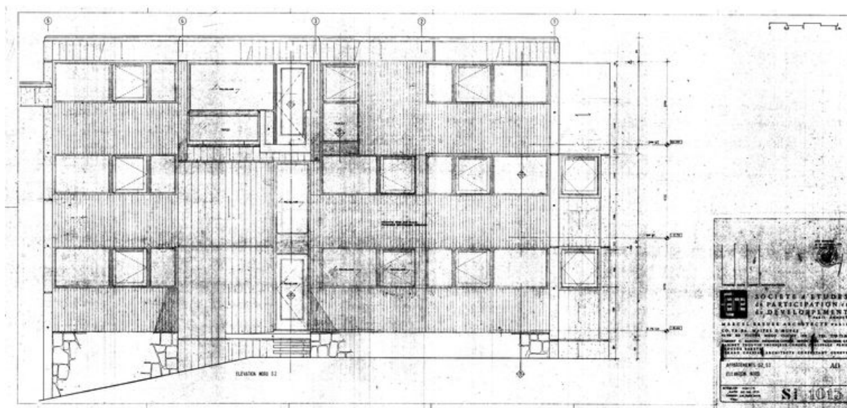
Appartements S2, S3. Elévation nord. Marcel Breuer, 30 mai 1975, modifié 14 août 1975 (AC Arâches-la-Frasse)
