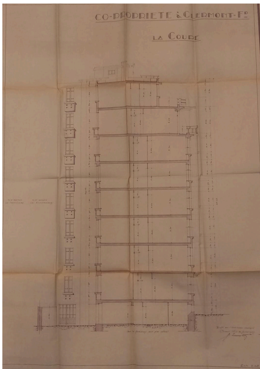
Coupe transversale
