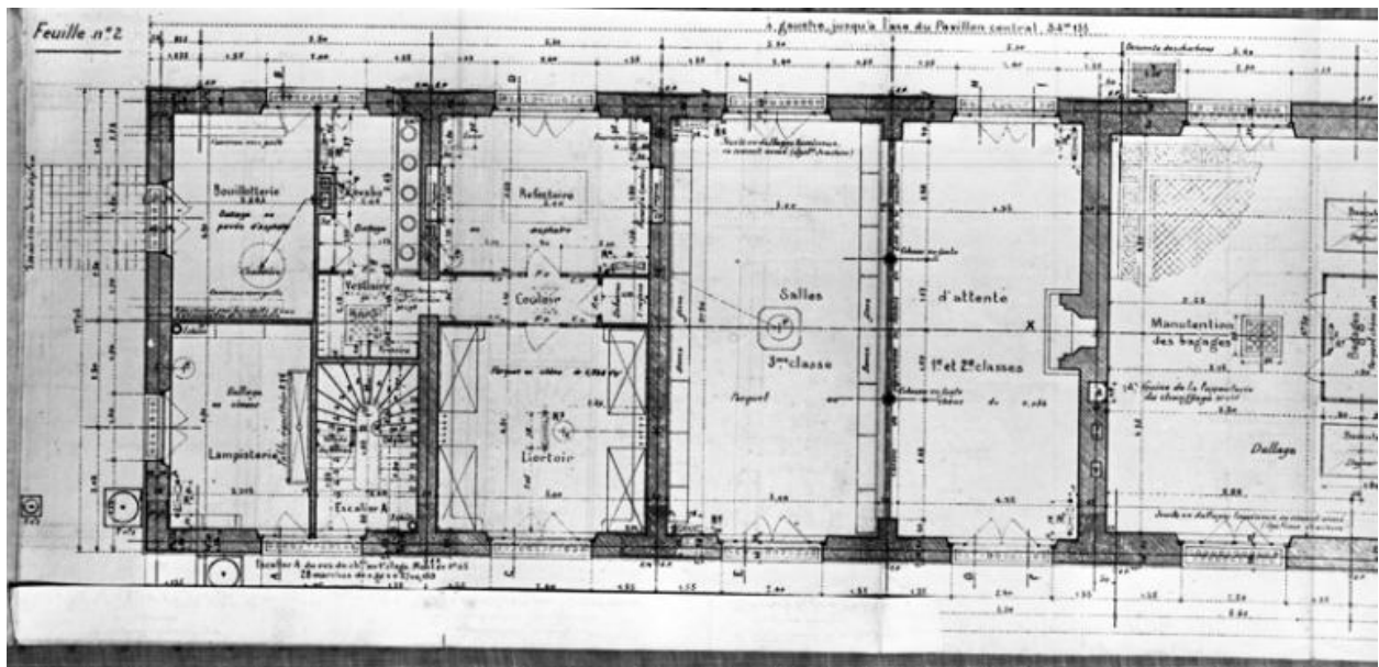
Gare de Châtel-Guyon. Bâtiment des voyageurs. Plan du rez-de-chaussée.
