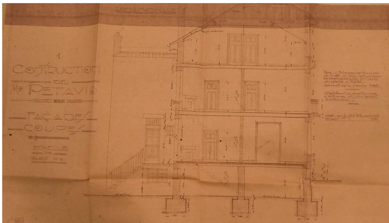
Coupe transversale du 23 boulevard Cote-Blatin
