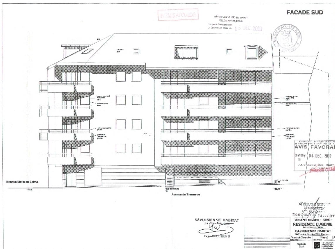
Façade sud
