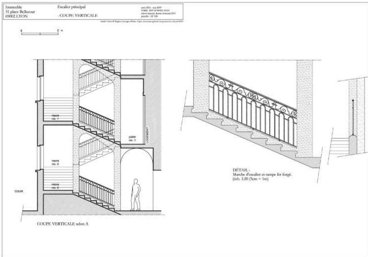
Relevé de l'escalier (Dess. A. Céréza, 2019)
