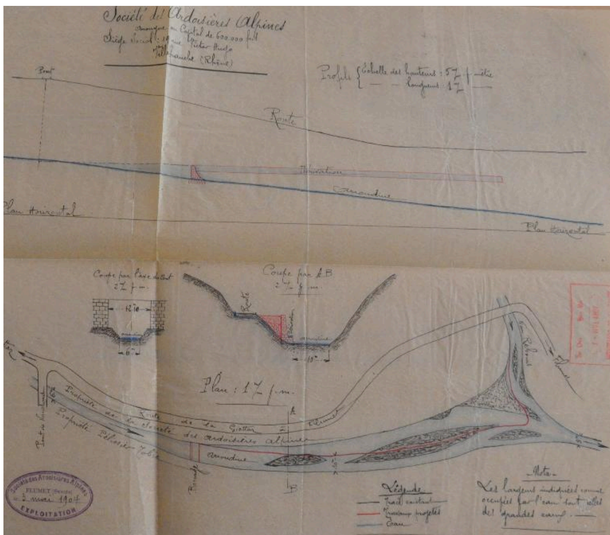
Projet de centrale de la Société des Ardoisières, 1904 (FR.AD073, 82S14).
