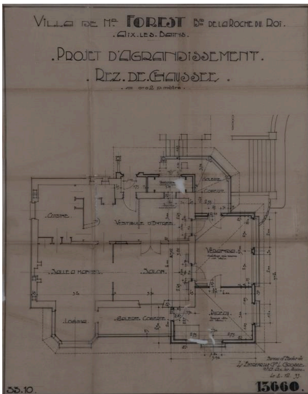
Plan du rez-de-terre, 1933
