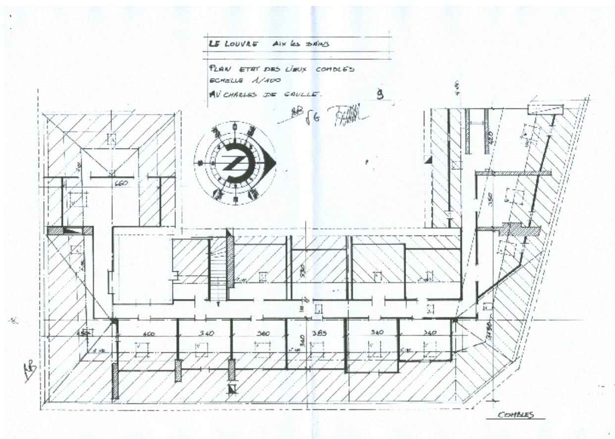
Plan des combles avant travaux
