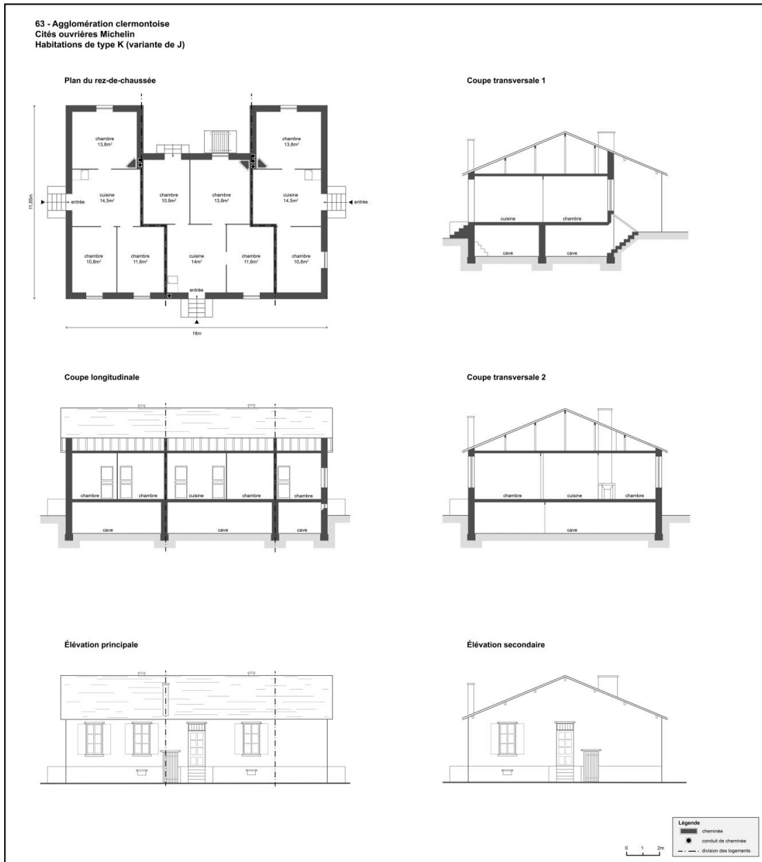
Plans, coupes, façades des habitations de type K (variante du type J)
