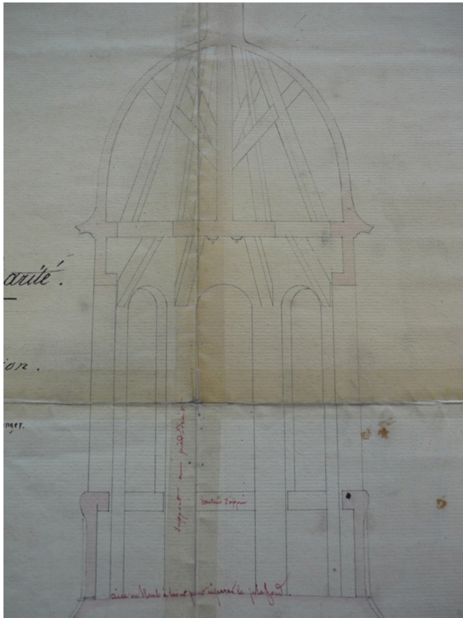
Projet de réparation du clocher, 1837 (détail du lanternon). Plan AC Lyon. Fonds des HCL ; 2OP691
