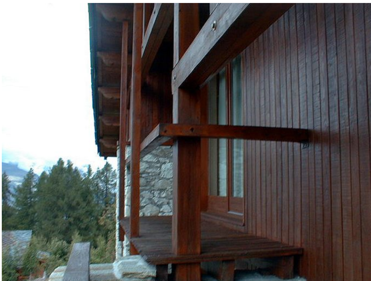
Détail d'une terrasse et du garde-corps
