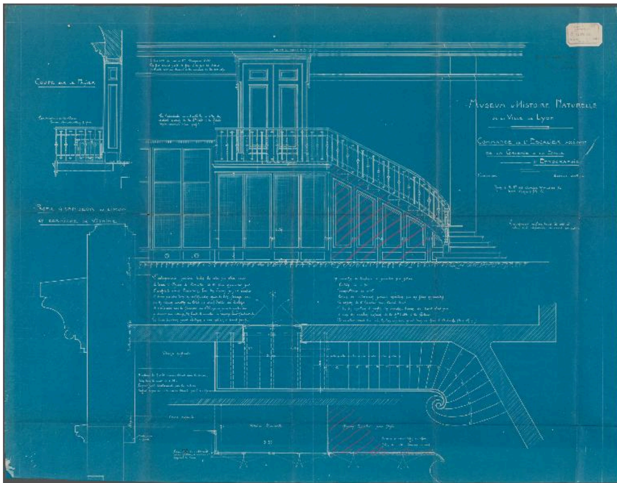
Muséum d'histoire naturelle : commande de l'escalier accédant de la galerie à la salle d'ethnographie, plan, coupe, élévation, profil, Tony Blein architecte, 22 janvier 1913. AC Lyon, 515 WP 6 2
