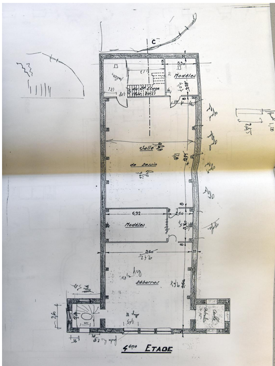
Plan du 4e étage : salle de dessin, non daté (AC Bourg-en-Bresse, 985 W 144)
