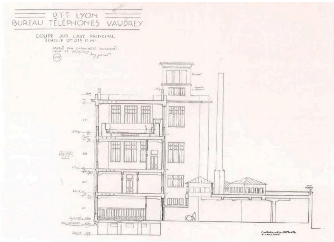
Coupe sur l'axe PTT Lyon Bureau téléphonique Vaudrey, Tony Garnier 1919 (Coll. MUTG)
