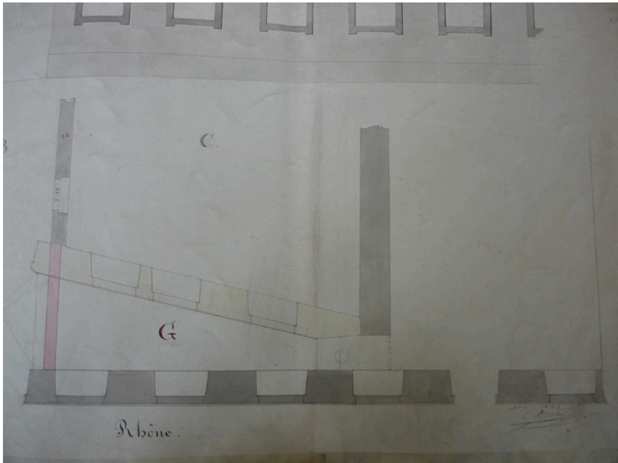
Elévation de la partie à construire pour l'achèvement de la façade sur le quai, 12 mars 1834 (détail de la coupe). Plan AC Lyon. Fonds des HCL ; 2OP680
