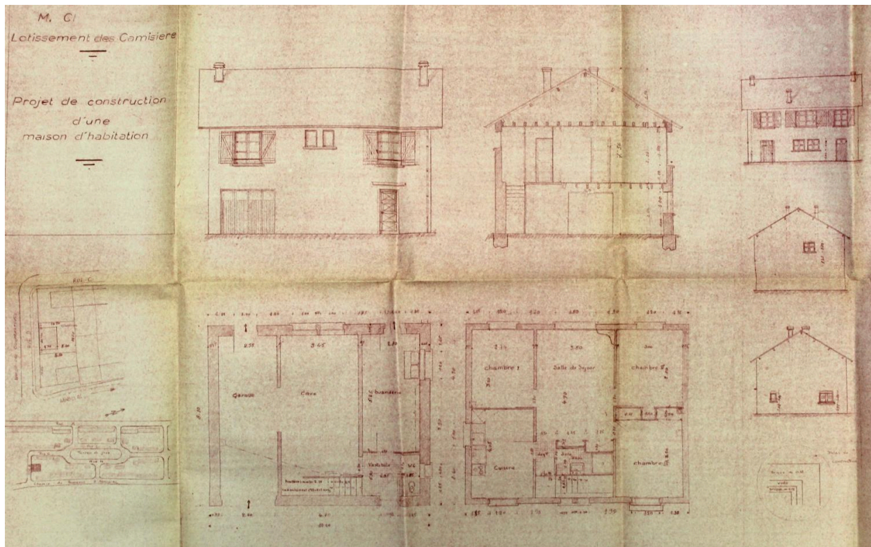
Aurillac, cité des Camisières, maisons n° 9 rue de la Doire, plan dérivé du plan-type des maisons HLR, n. d., vers novembre 1954, non signé, attribué à l'architecte Jacques Porcher (Archives municipales d'Aurillac, 135 W 46, permis de construire n° 1465).
