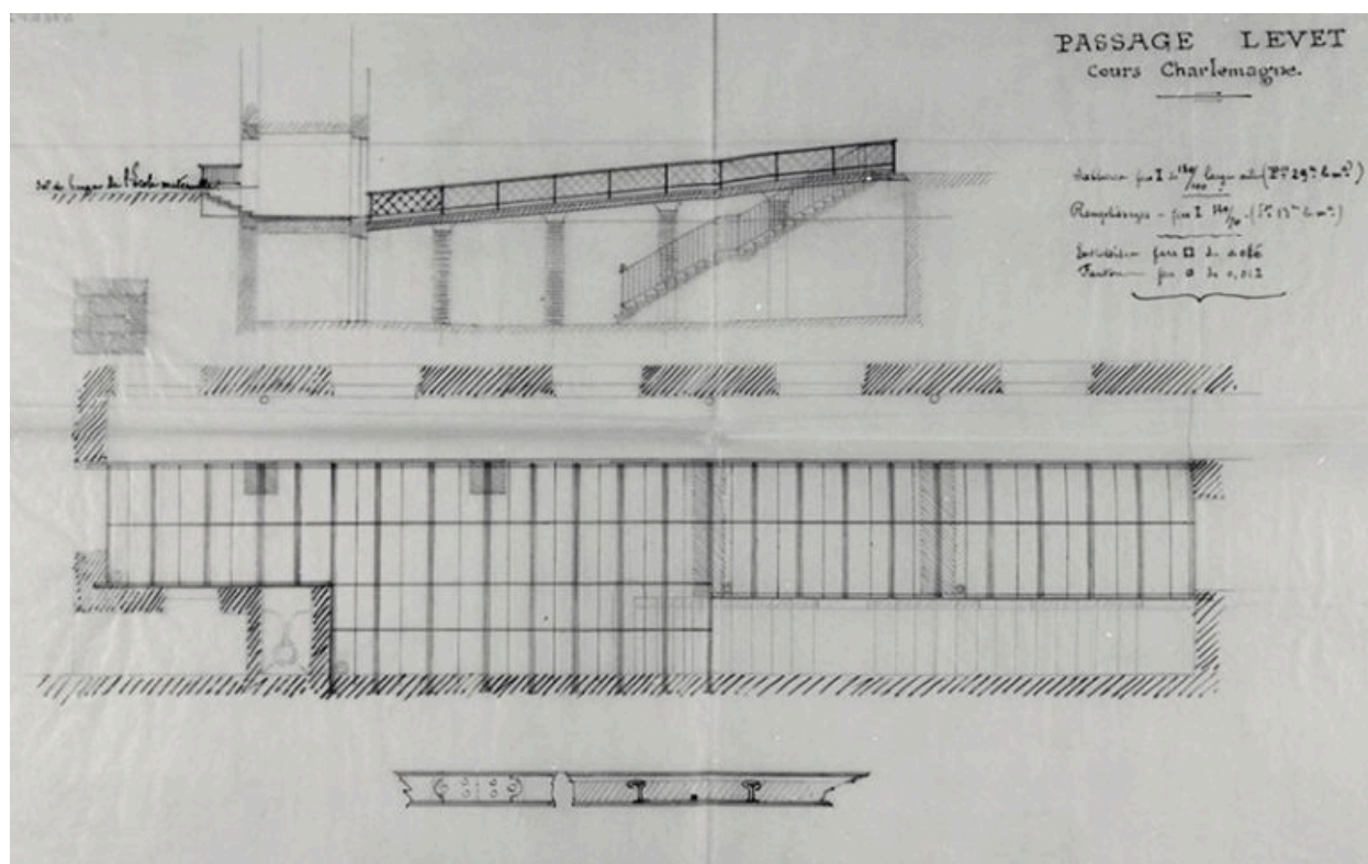
Passage Levet reliant l'école au cours Charlemagne : plan et élévation
