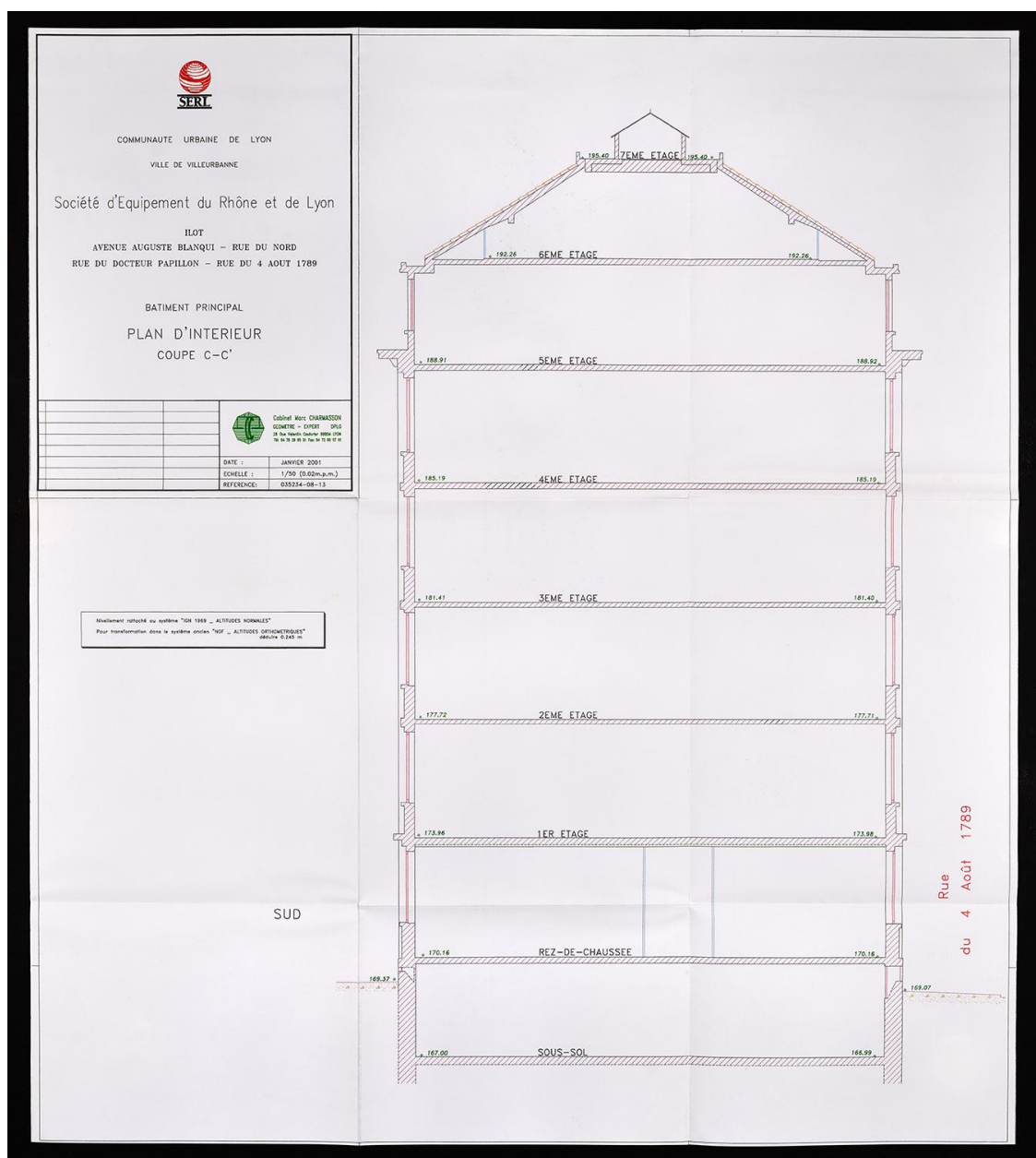
Coupe bâtiment principal (SERL)
