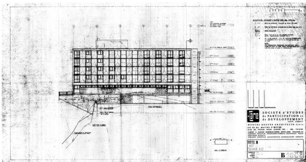
Hôtel B. Elévation est. Marcel Breuer architecte, 10 septembre 1966 (AC Arâches-la-Frasse)
