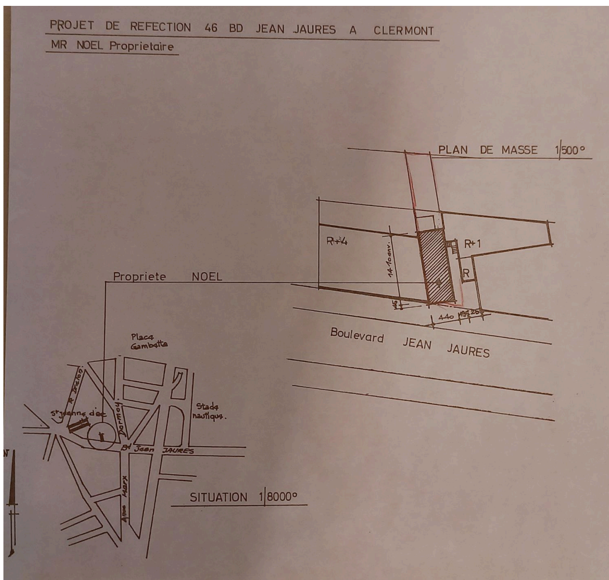
Plan de masse et de situation (rénovation immeuble, 1968)
