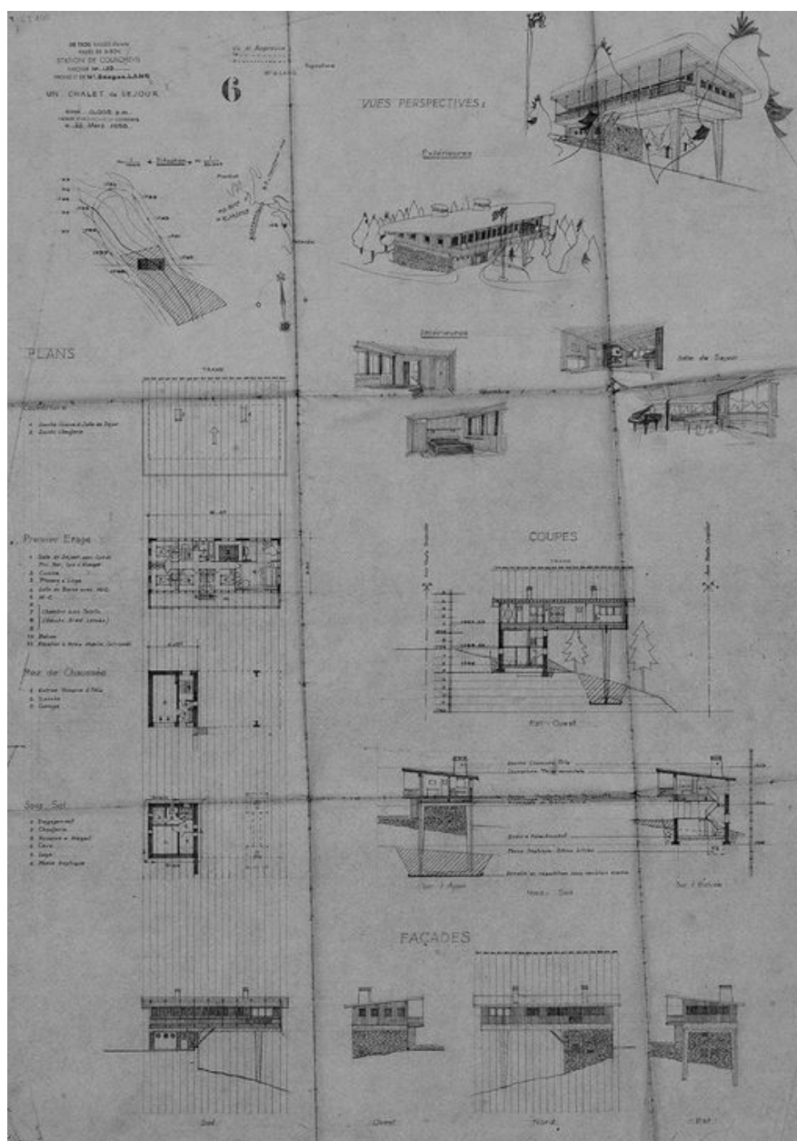
Un chalet de séjour. Plans, coupes, élévations / Atelier d'Architecture de Courchevel, 22 mars 1950 (AD Savoie. 6J 100)
