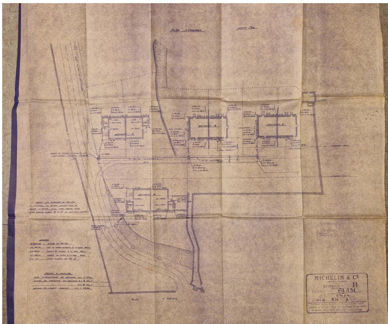
Projet de cité "employés" : plan d'implantation, 1929.
