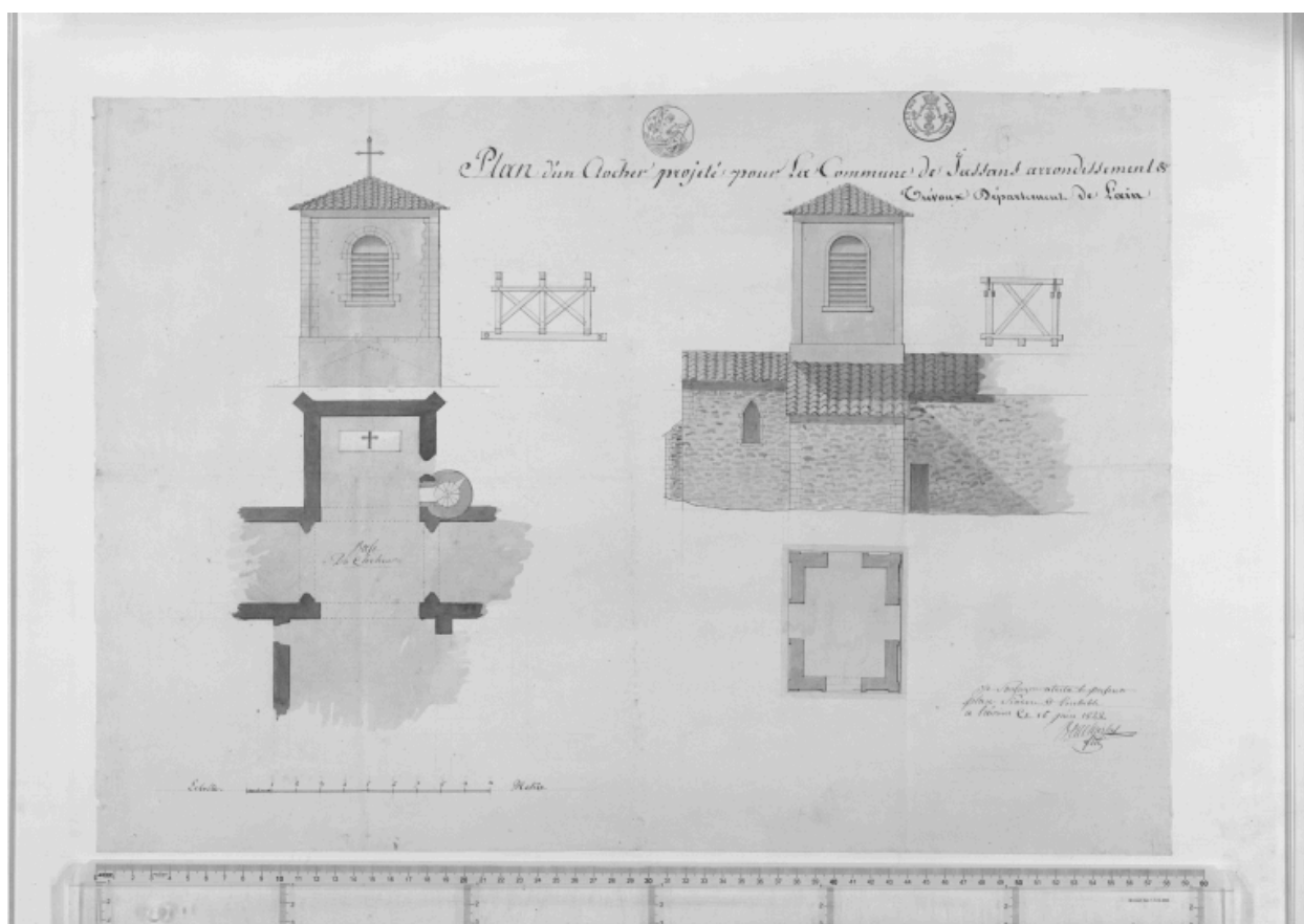
Plan d'un clocher projeté pour la commune de Jassans..., par Boucharlat fils, 16 juin 1822.
