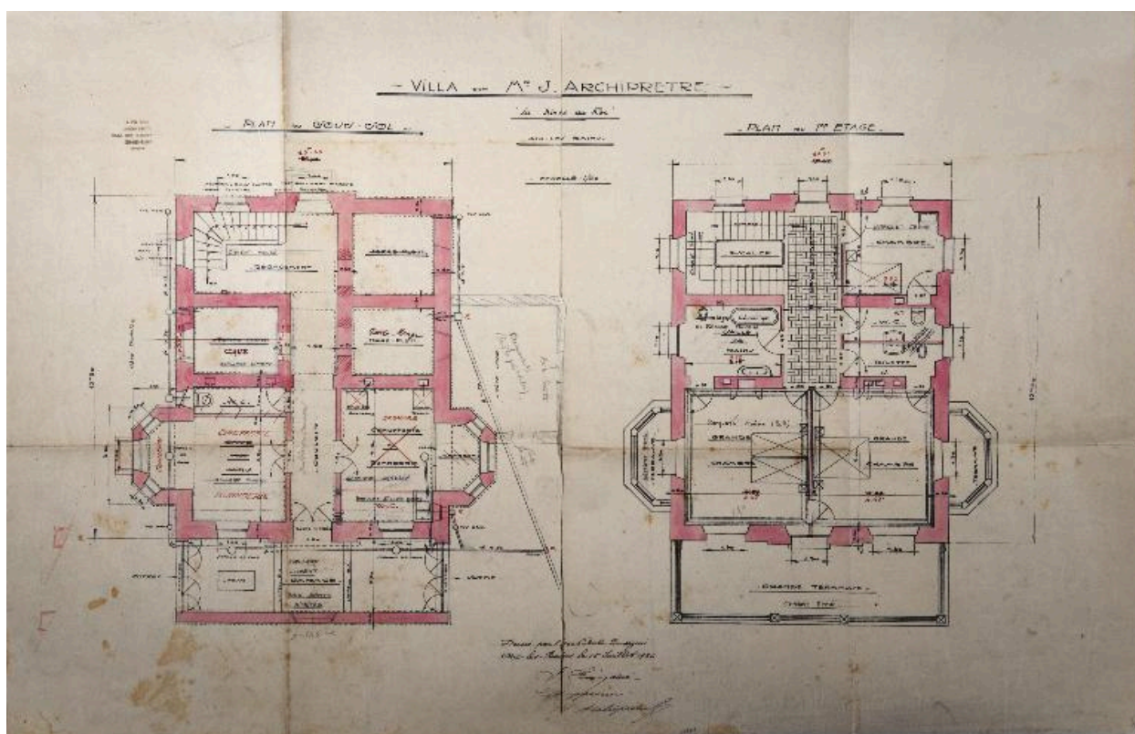
Plans du sous-sol et du 1er étage, 1926
