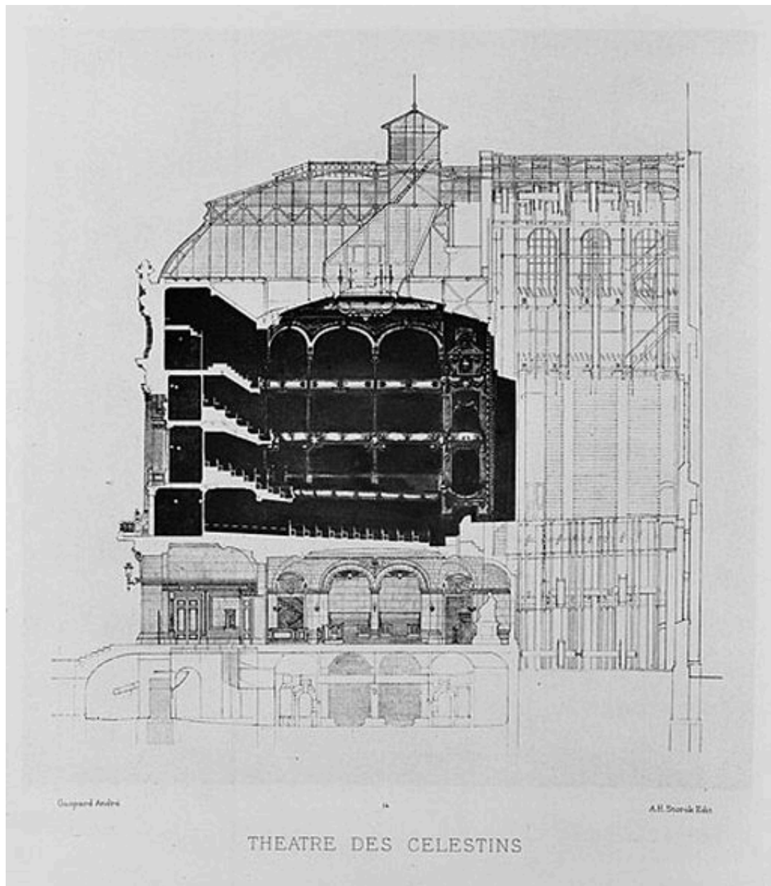
Théâtre de Gaspard André : Théâtre des Célestins [Coupe], estampe dans L'Oeuvre de Gaspard André, Lyon : A. Storck, 1898, pl. 14
