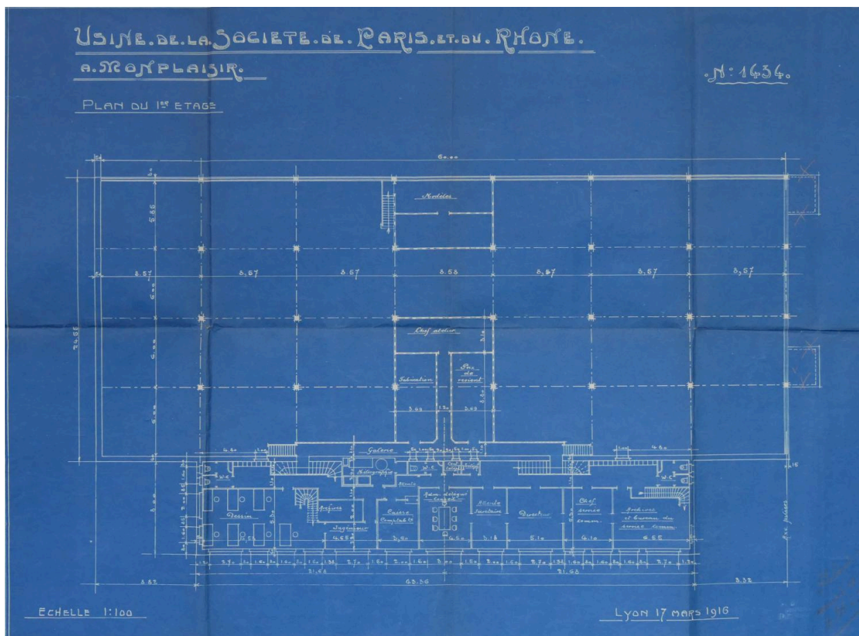
Plan du 1er étage (AC Lyon 314w574, 1916)
