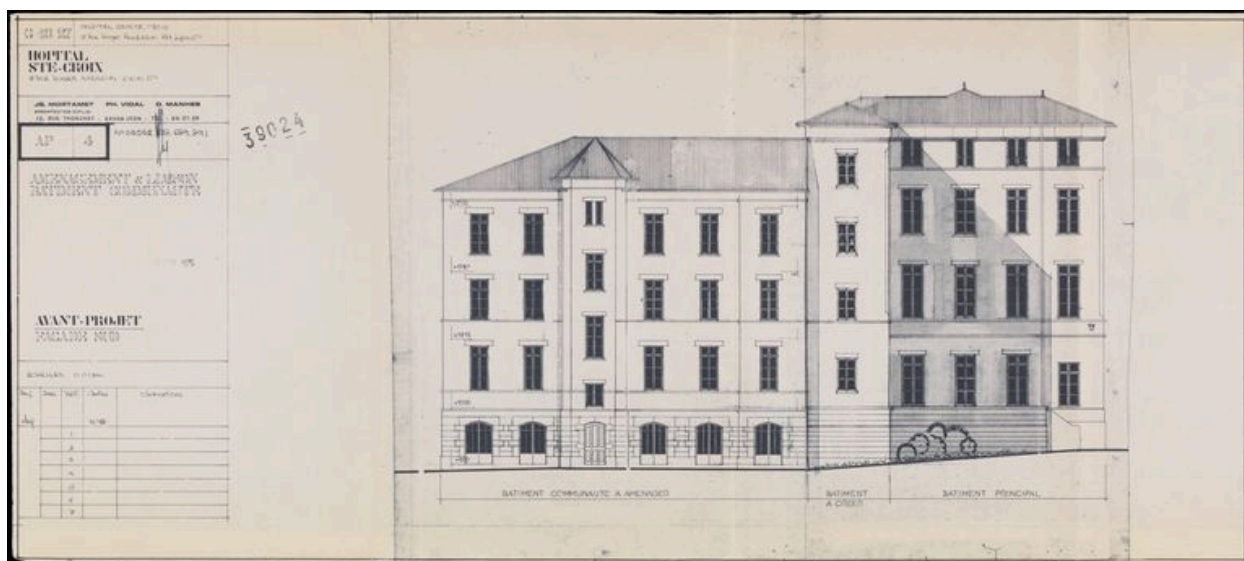
Elévations sud : avant-projet de l'agence Mortamet (c. 1979) (Arch. mun. Lyon, 905 WP_10, Agence Mortamet, Vidal, Manhes, tirage d'architecte).
