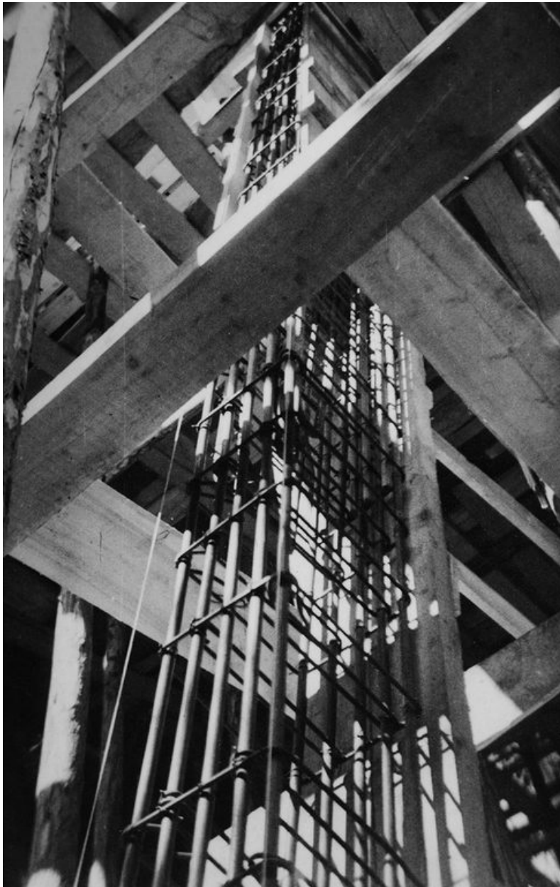
Le chalet en construction. L'ossature métallique. Photogr. Denys Pradelle, [1950] (AD Savoie. 6J 100)
