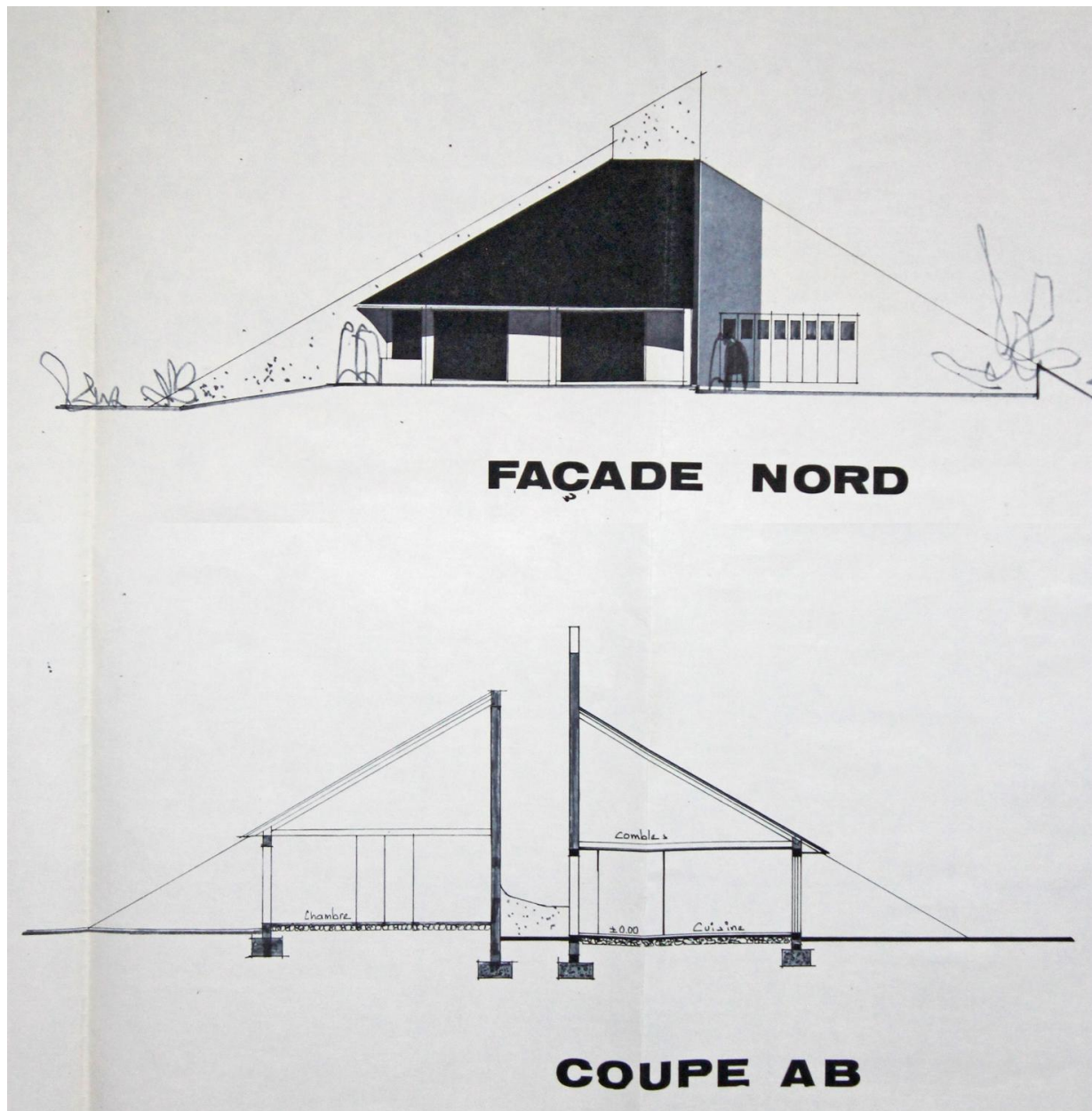
Orcines, la maison Ver.*, façade nord et coupe A-B, octobre 1970, Jean-Claude Breuil architecte (archives communales d'Orcines).
