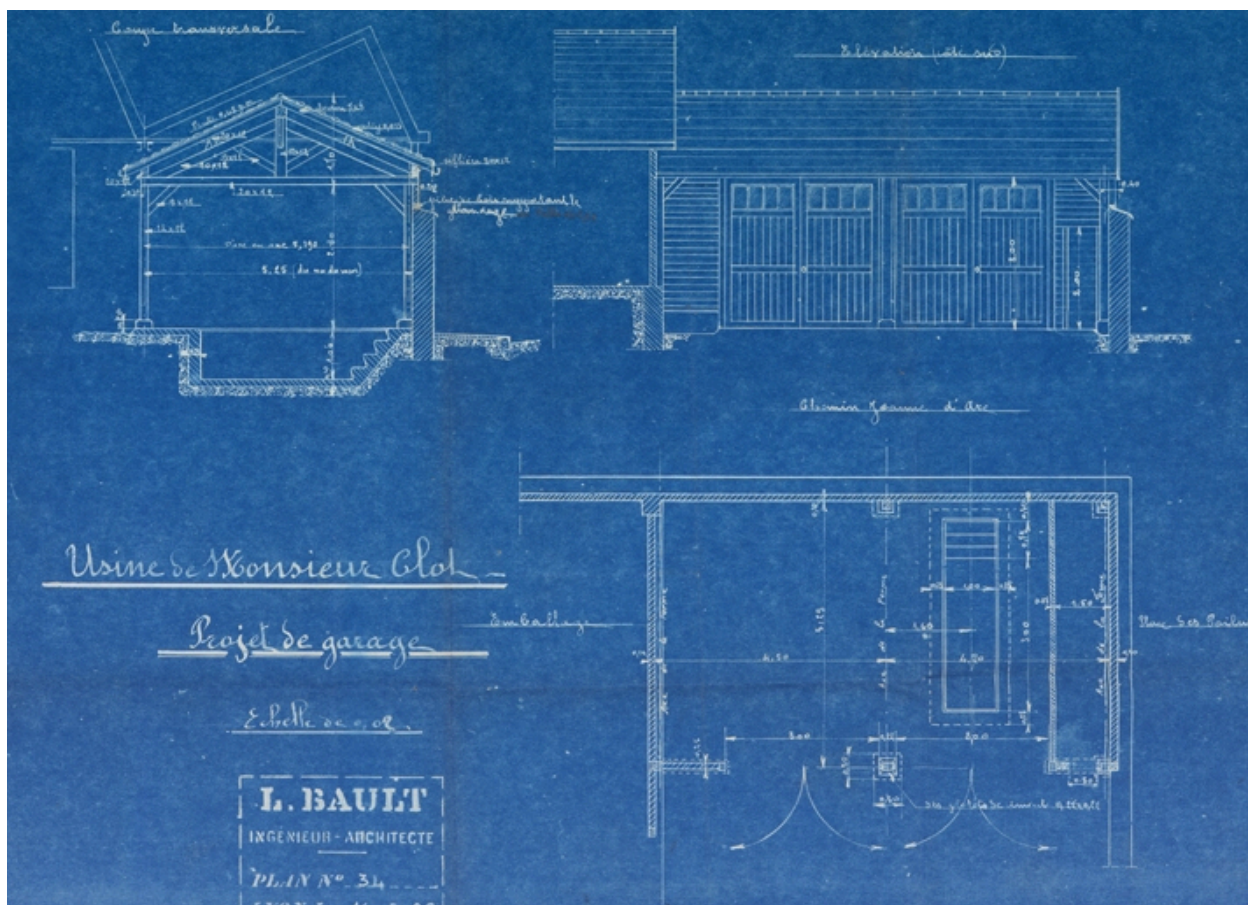
AC Lyon : 323 WP 041 PCA n°673, plan, coupe, élévation d'un garage pour M. Clot pas M. Bault, 1922
