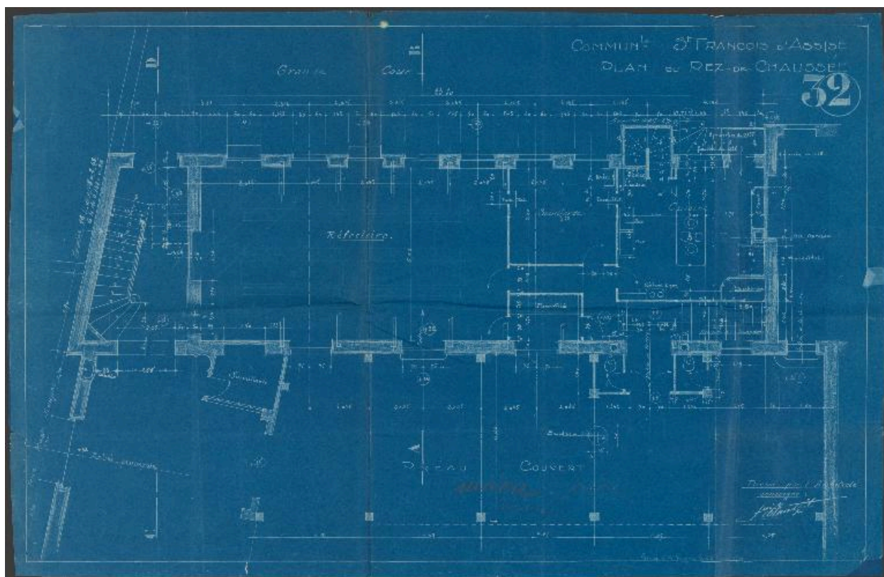
Communauté Saint-François d'Assise : plan du rez-de-chaussée / François Roux-Spitz architecte. 1927 (AC Lyon 344 W 732)
