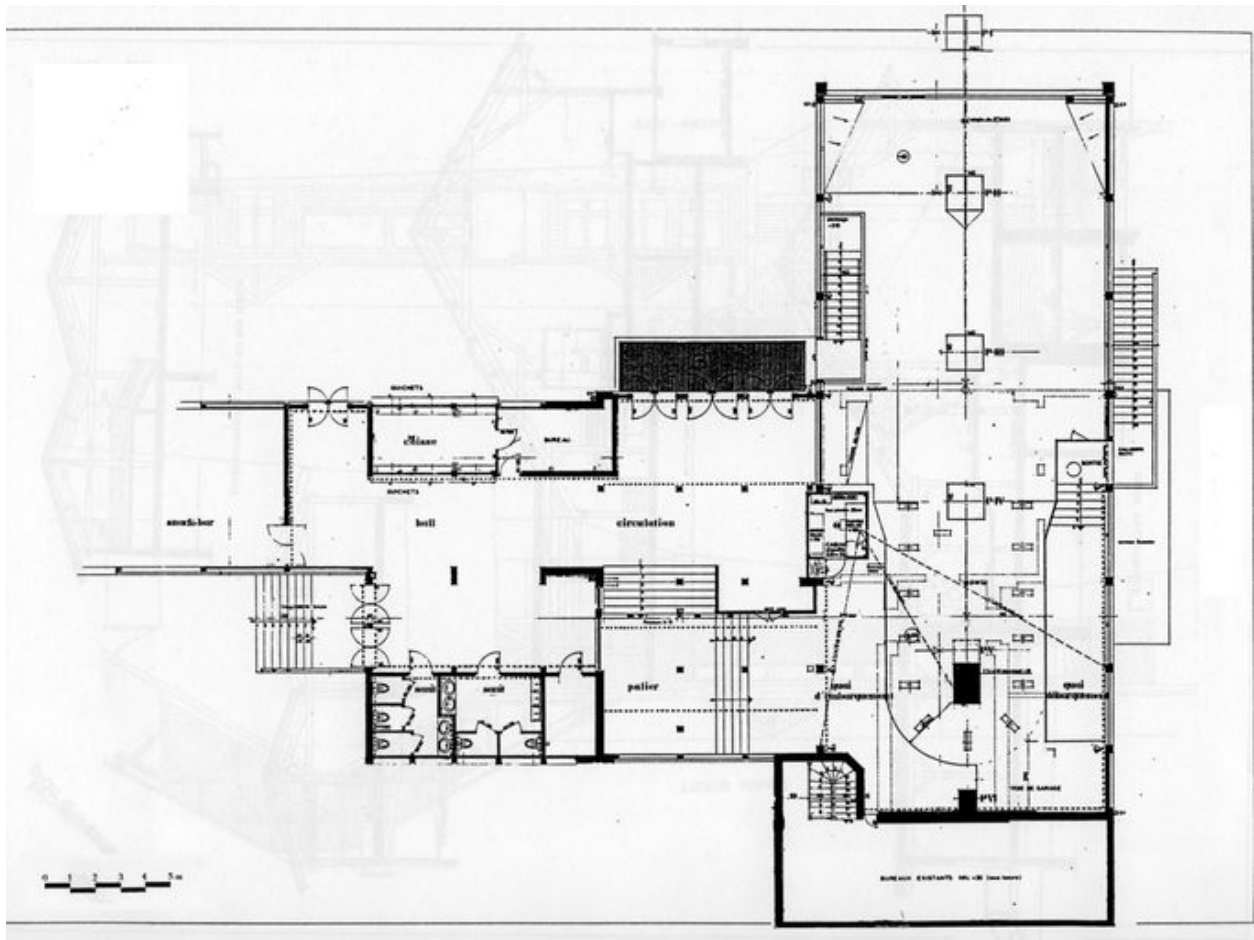
Gare inférieure. Plan au niveau des quais / [Pierre Duclos, 1985]
