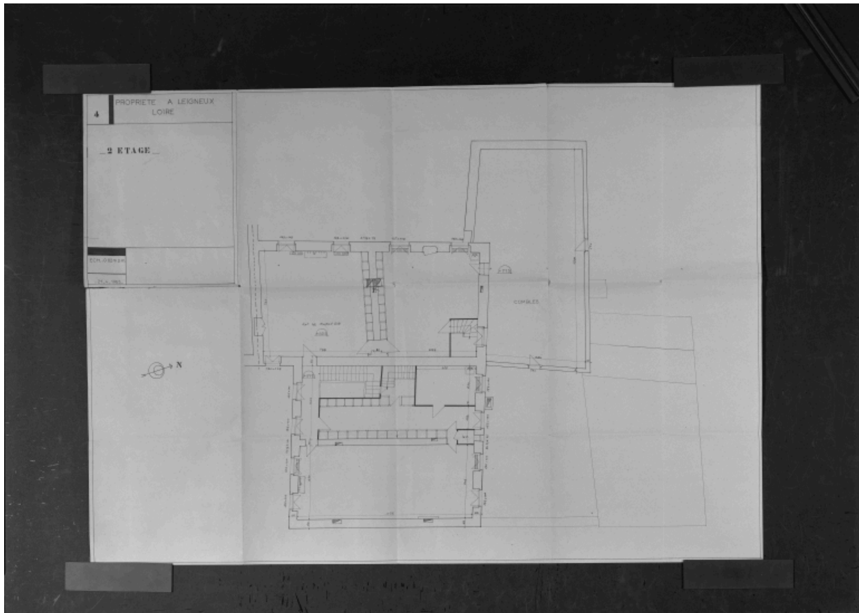
Propriété à Leigneux. Loire. 2 étage. Ech. 0,02 m. p. m." Plan du 2e étage.
