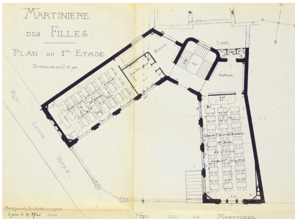
Plan du 1er étage. 1:100. 2 mai 1904. Document figuré. Coupe. Archives du Lycée de la Martinière (intendance Augustins). non coté
