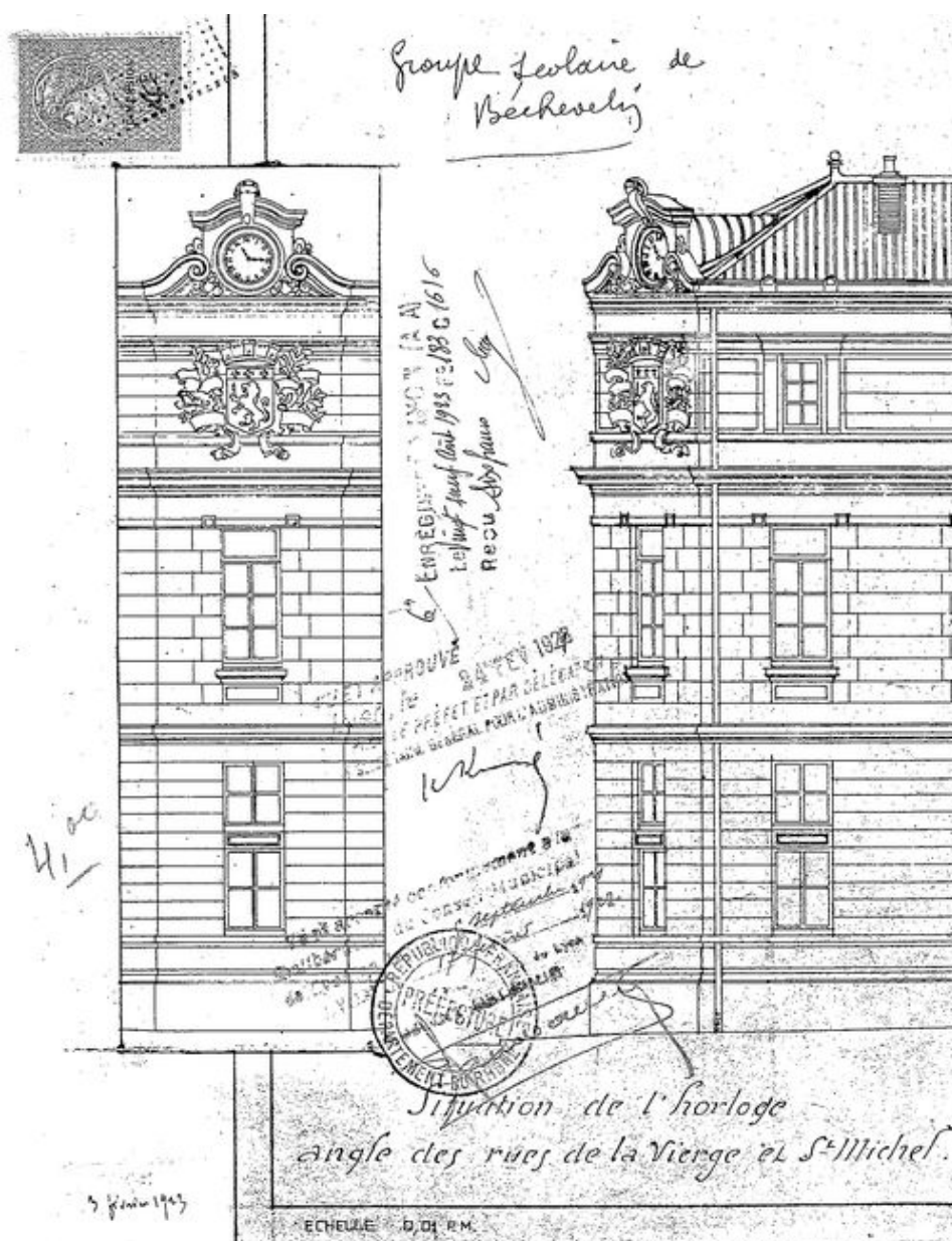
Dessin de la travée d'angle des rues Gilbert-Dru et Saint-Michel, 1923
